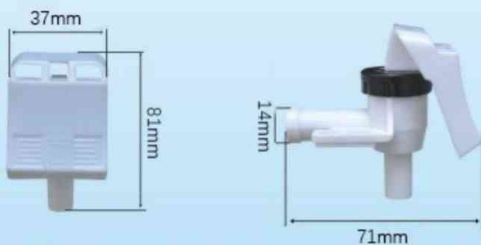
TY-097 4孔中心距30x11.5mm
