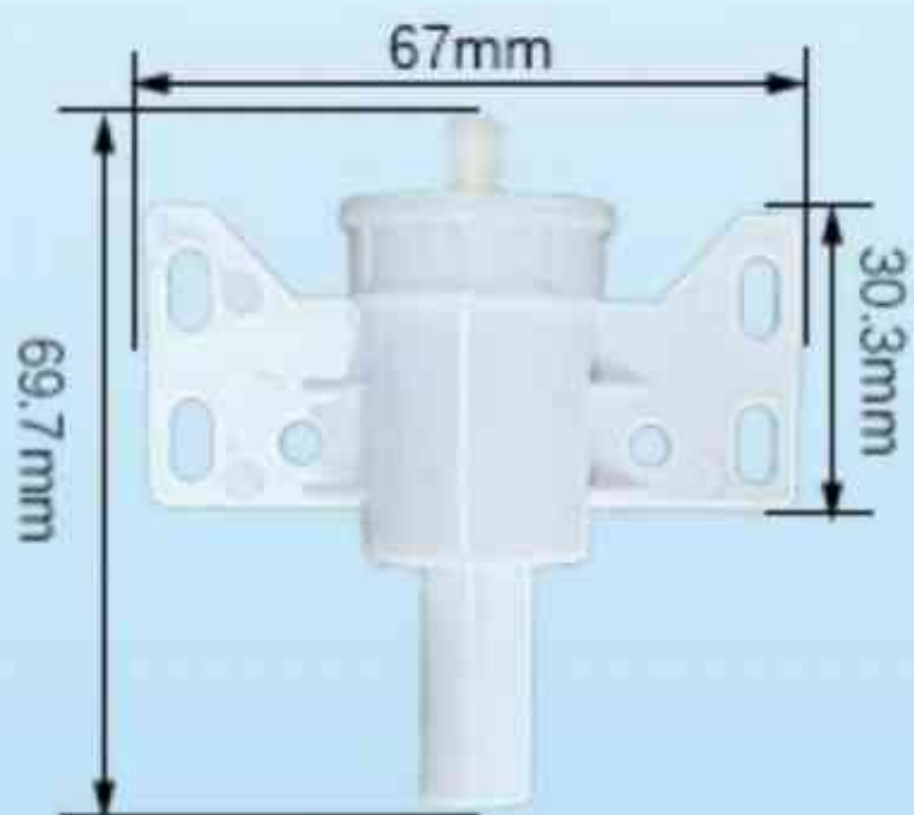
TY-175
