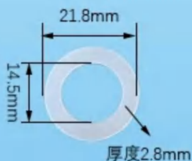
118硅胶平垫
