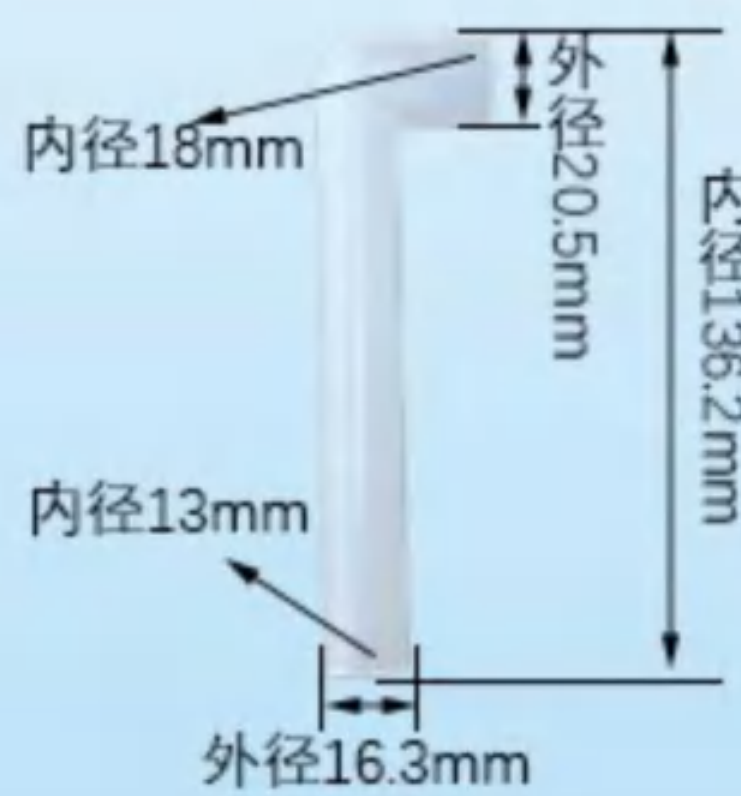
大头弯管
