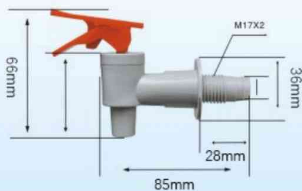
TY-065防烫型 Male
