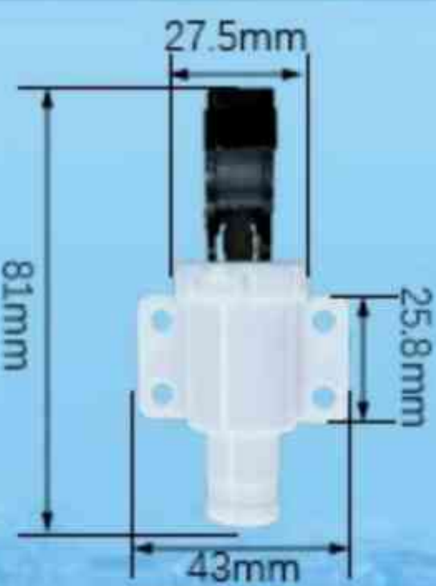
TY-171-1
