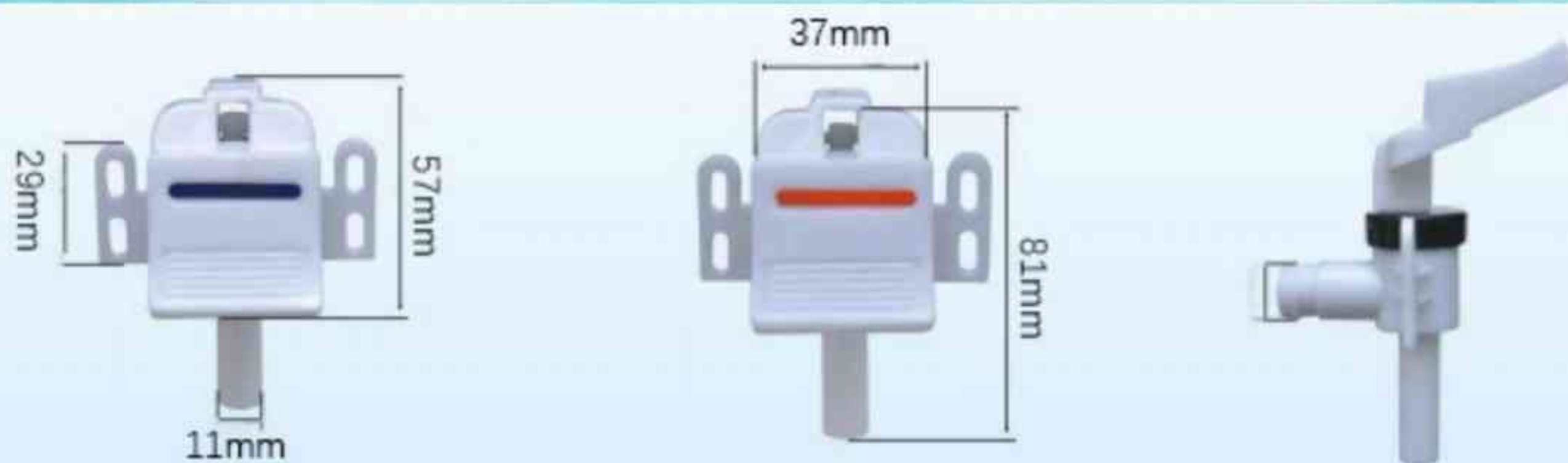
TY-096 4孔中心距61x15mm
